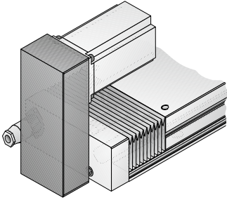
Anbauvariante zum Verschiebeteil Qi Assembly type to the shifting element Qi i = 1:1
