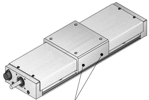
beidseitig Schmiernippel für Kugelbüchsen Grease nipple for ball bushings on both sides
