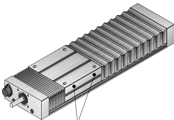
beidseitig Schmiernippel für Kugelbüchsen Grease nipple for ball bushings on both sides
