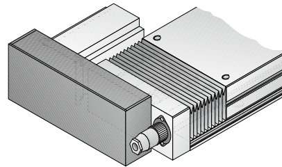
Anbauvariante nach links, Verschiebeteil oben Sl Assembly type left, shifting element above Sl i = 1:1
